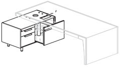
SX CX2960 (DX) L110,2 P57 H61,6 CX2961 (SX) L110,2 P57 H61,6
