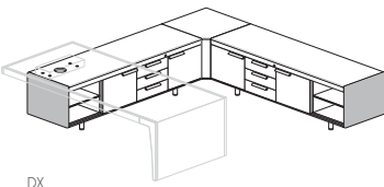
DX CX2932 (DX) L256,4 P256,4 H61,6 CX2931 (SX) L256,4 P256,4 H61,6
