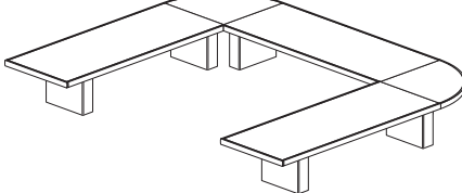
CX1638 L387,1 P299,4 H75 CX1641 L411,1 P323,4 H75 CX1644 L437,1 P349,4 H75
