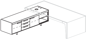
SX CX2906 (DX) L193,5 P57 H61,6 CX2905 (SX) L193,5 P57 H61,6
