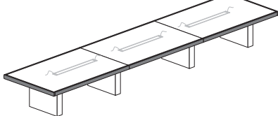
CX1653P L540,7 P121,7 H75 CX1670P L708,7 P121,7 H75
