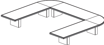
CX1638P L387,1 P299,4 H75 CX1641P L411,1 P323,4 H75 CX1644P L437,1 P349,4 H75
