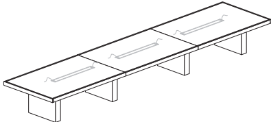
CX1653 L540,7 P121,7 H75 CX1670 L708,7 P121,7 H75
